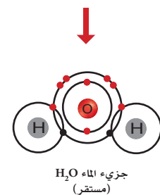
الشكل ٦ ب الرابطة التساهمية القطبية في جزيء الماء H_2O .
