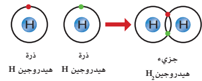
الشكل ٦ أ الرابطة التساهمية غير القطبية في جزيء الهيدروجين H_2 .
