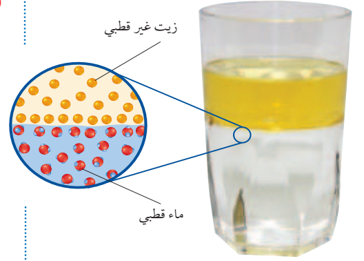
الشكل ٩ الماء والزيت لا يختلطان؛ لأن جزيئات الماء قطبية، وجزيئات الزيت غير قطبية.
